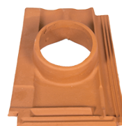
D025 Douille Ø 130 3,391 kg
