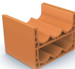
CASBOUMER (*) casier merlot 24 kg - 36 bouteilles au m 2
