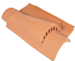
CH12 Chatière 3,508 kg
