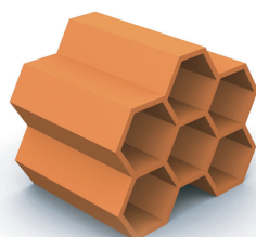
CASBOU6T (*) casier 6 bouteilles 15,2 kg - 36 bouteilles au m 2
