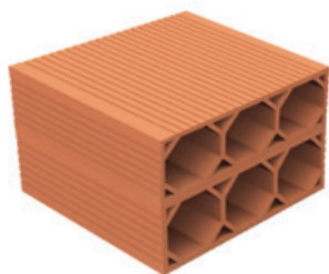
CASBOU3TX2 (*) 2 casiers 3 bouteilles 18,6 kg - 96 bouteilles au m 2
