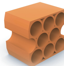
CASBOU9T (*) casier 9 bouteilles 16,5 kg - 36 bouteilles au m 2
