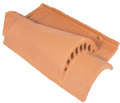
CH05 Chatière 4,4 kg
